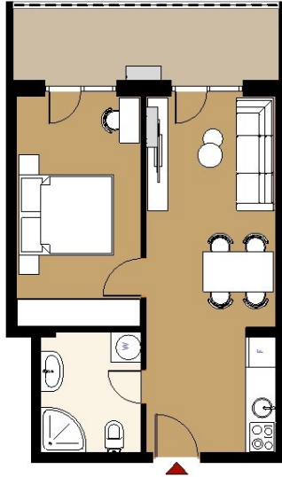
2D OSNOVA
